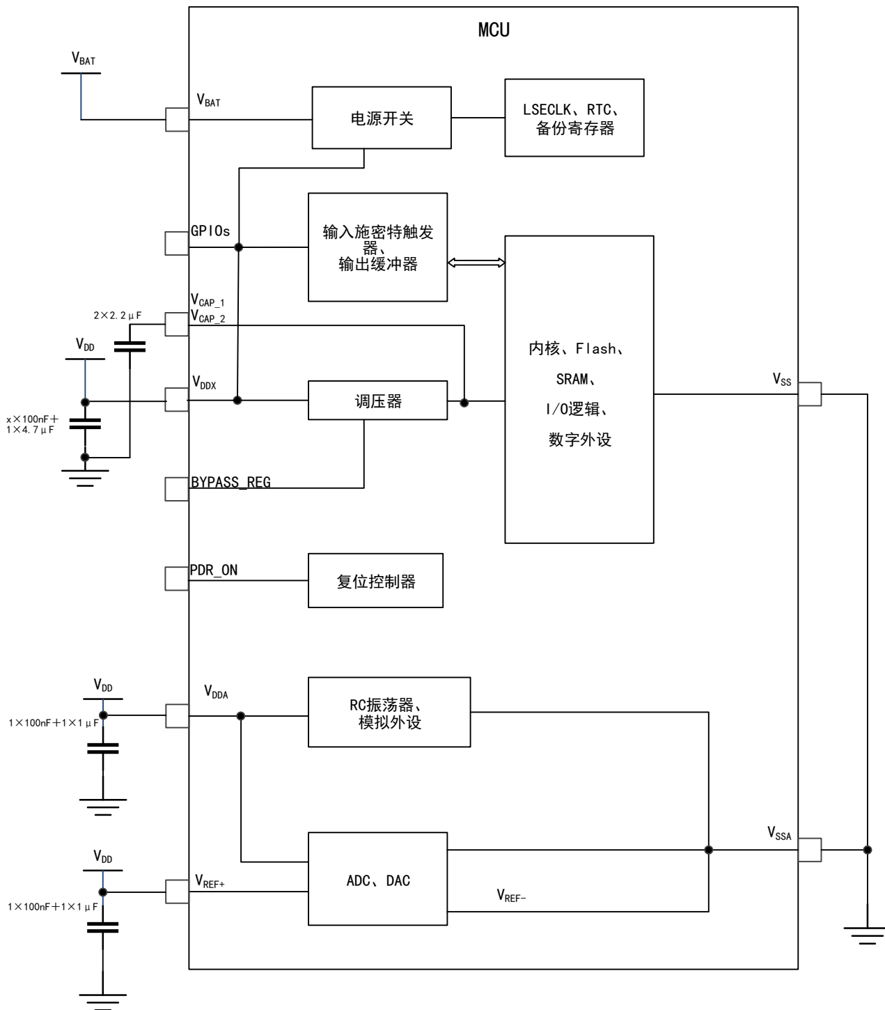
图 5 电源方案
